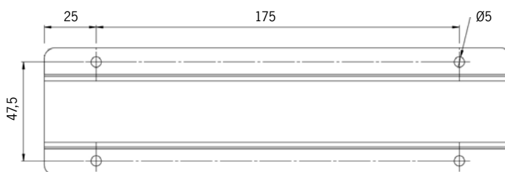
Fästbygel ramp 1027088
